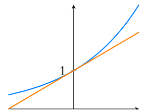
FIGURE 1.3– L'exponentielle et sa tangente en 0.
