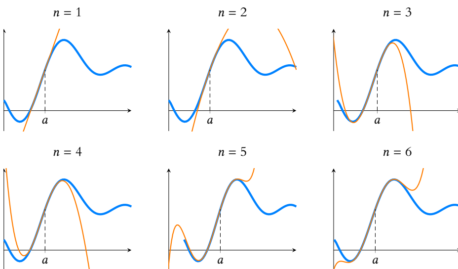
FIGURE 22.1 – Les premiers développements limités d'une fonction f . On constate qu'au voisinage de a , f est très bien approximée par ses développements limités, et que plus n est grand, plus l'approximation reste correcte «loin» de a .
